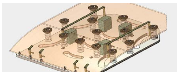
13 molas dinâmicas especificamente adaptadas para os saltos
