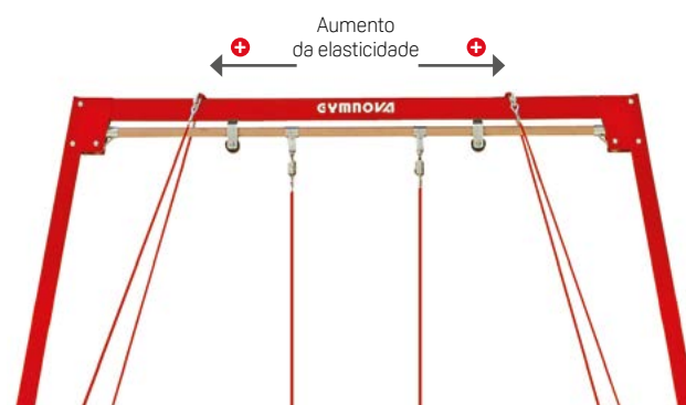
Regulação da elasticidade
