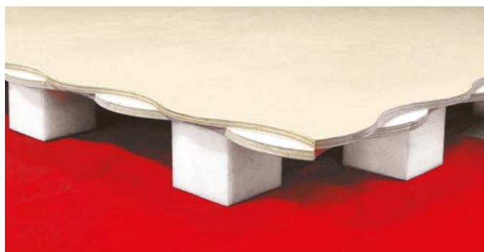
Detalhe das placas com perímetro ondulado
