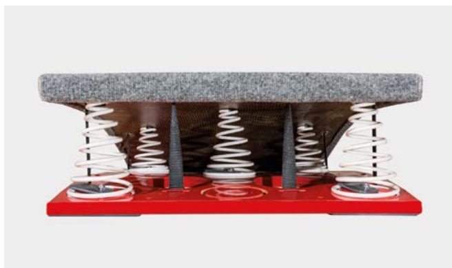
Molas cónicas
