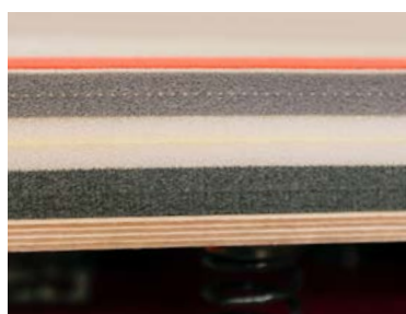
Complexo de espuma com 56 mm de espessura
