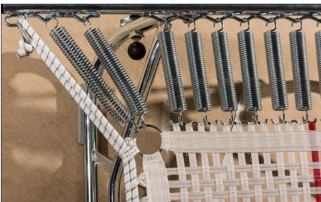
Tensada mediante 32 muelles
