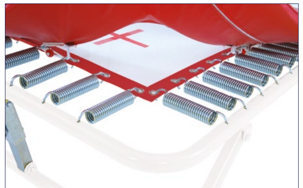
34 muelles galvanizados conectados a la cama elástica de PVC
